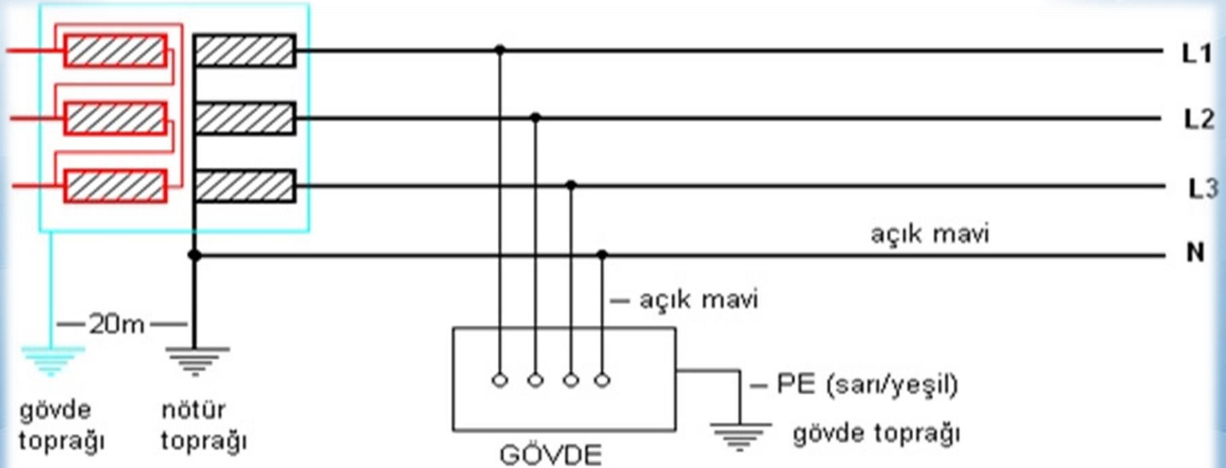
TT ELEKTRİK ŞEBEKESİ TOPRAK YAPISI
