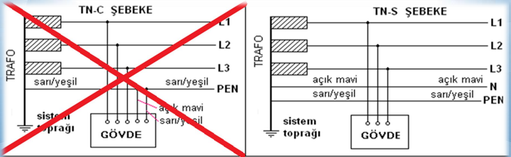
TN ELEKTRİK ŞEBEKESİ YAPISI (TN-C ve TN-S)
